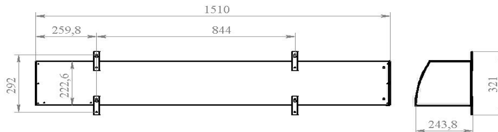
Рис. №1 Габаритные и установочные размеры завес T307E15, T309E15 и T314E15.
